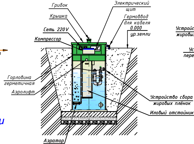
Разрез В-В
