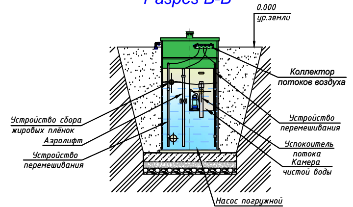
Разрез Б-Б
